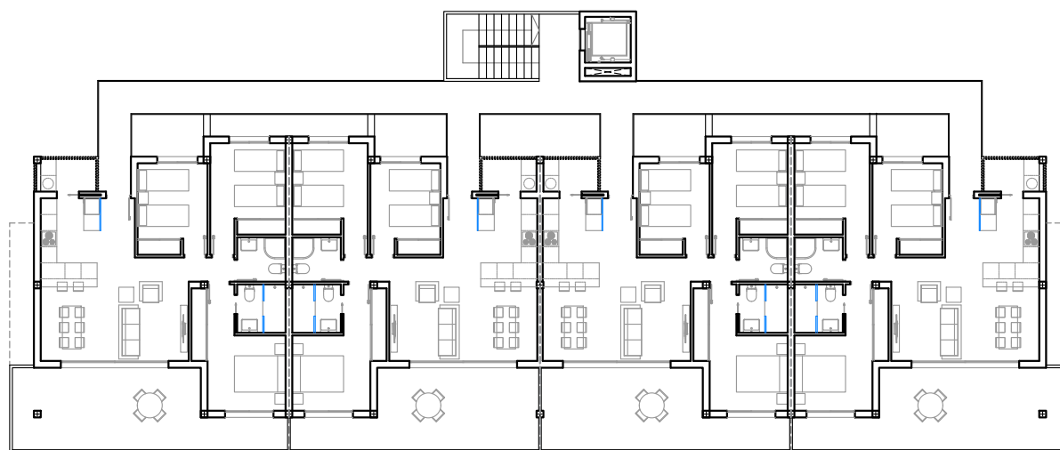
PLANTA PRIMERA
