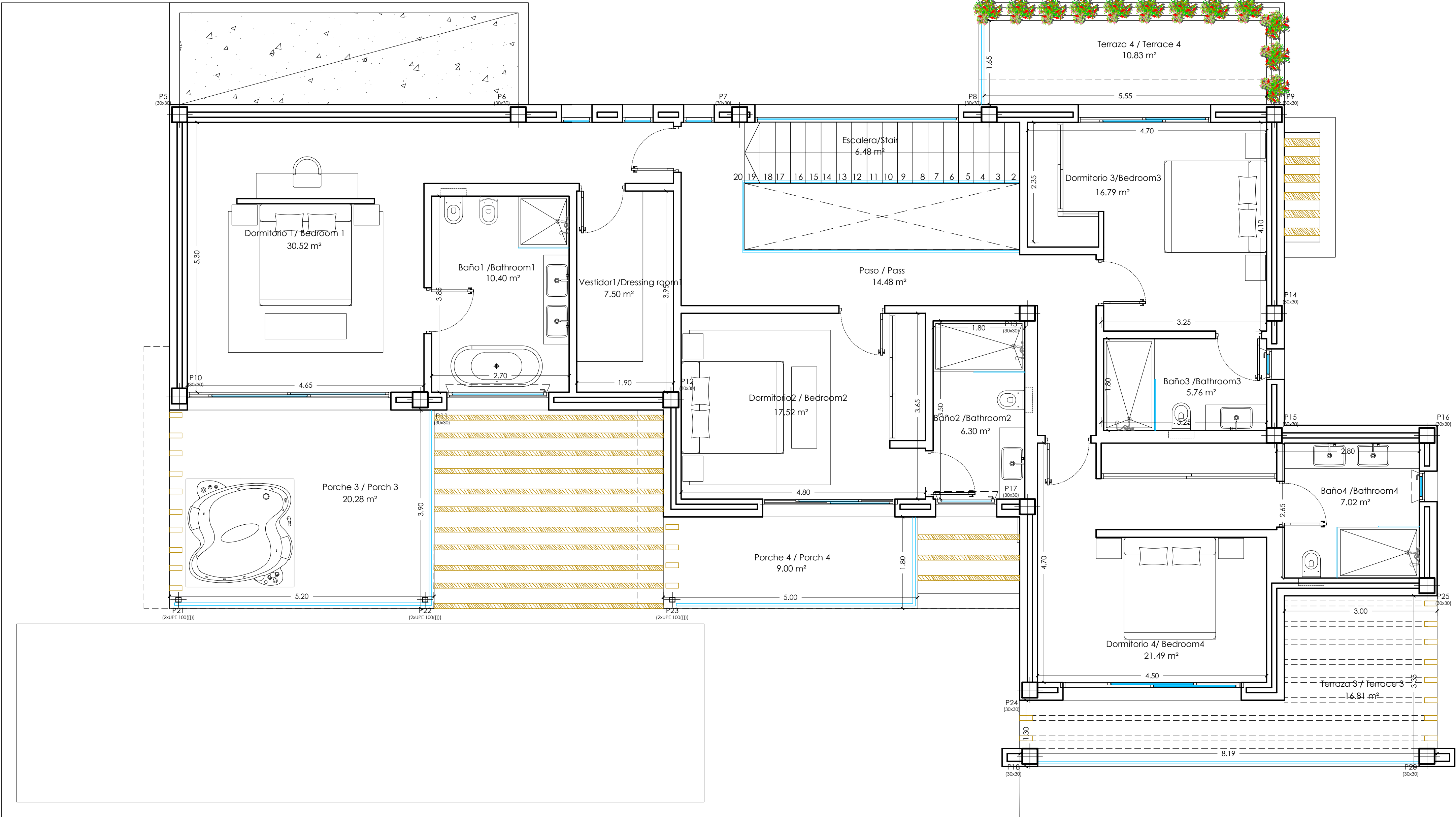
Planta Alta 185.77 m²
