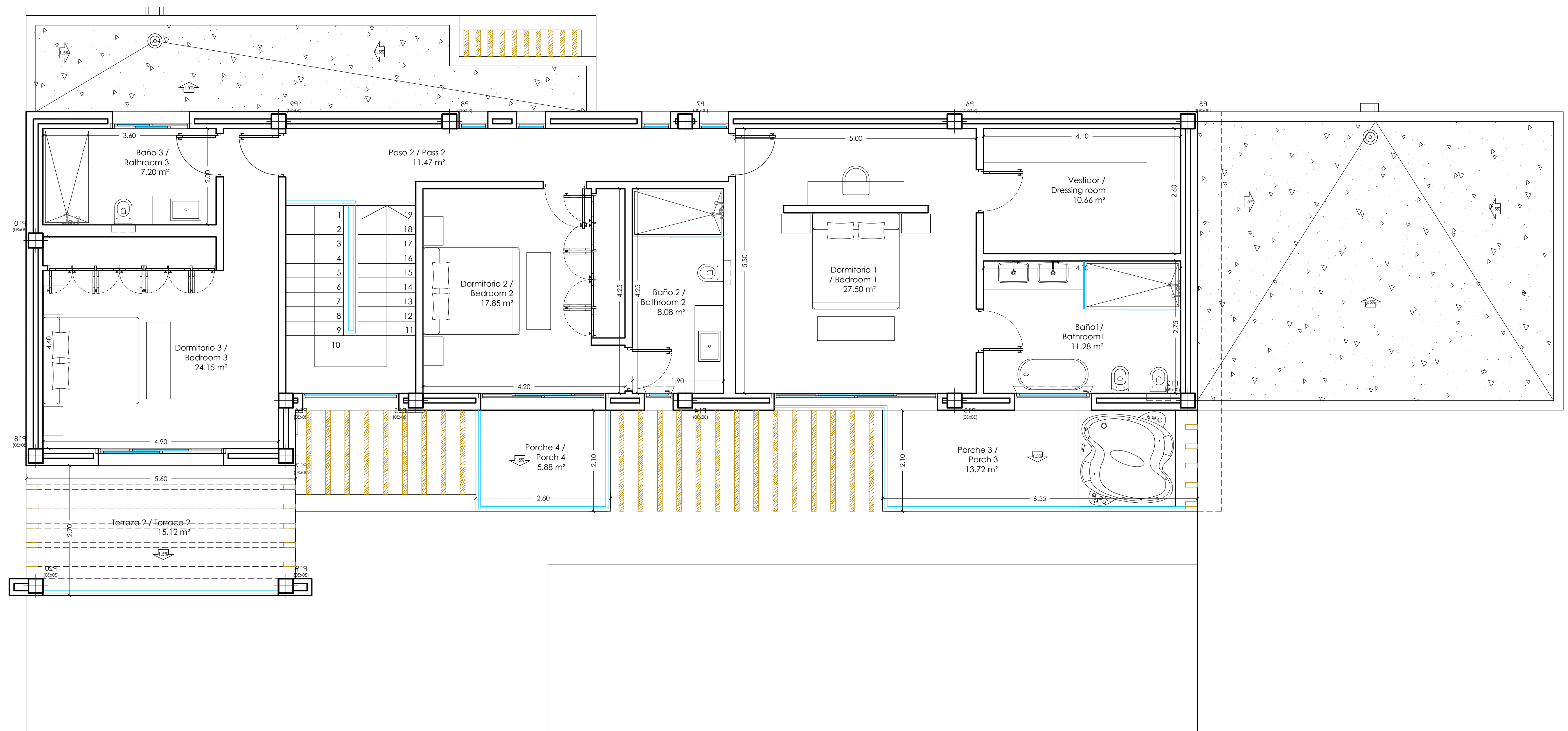
Planta Alta 157.41 m²
