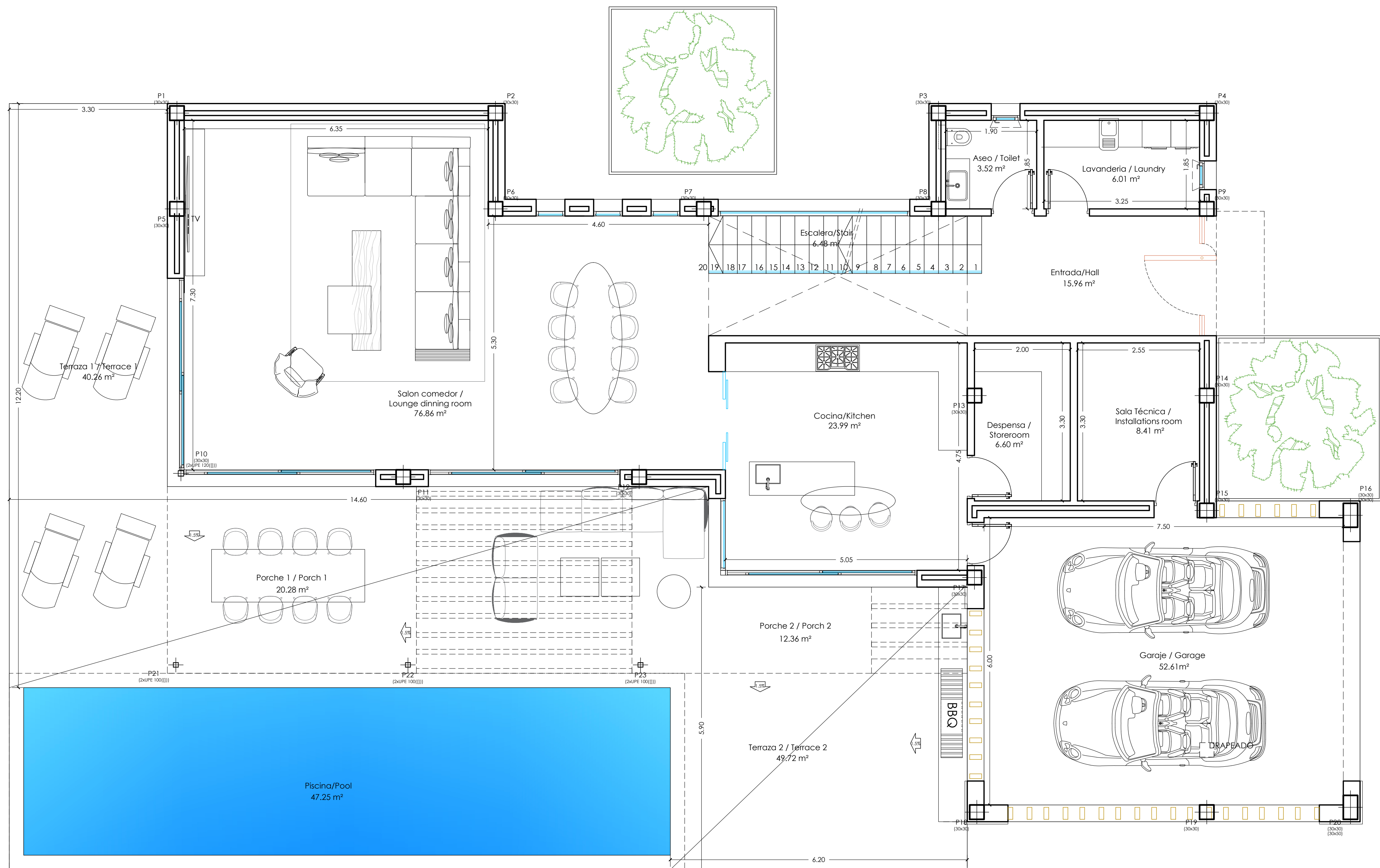
Planta Baja 172.72 m²
