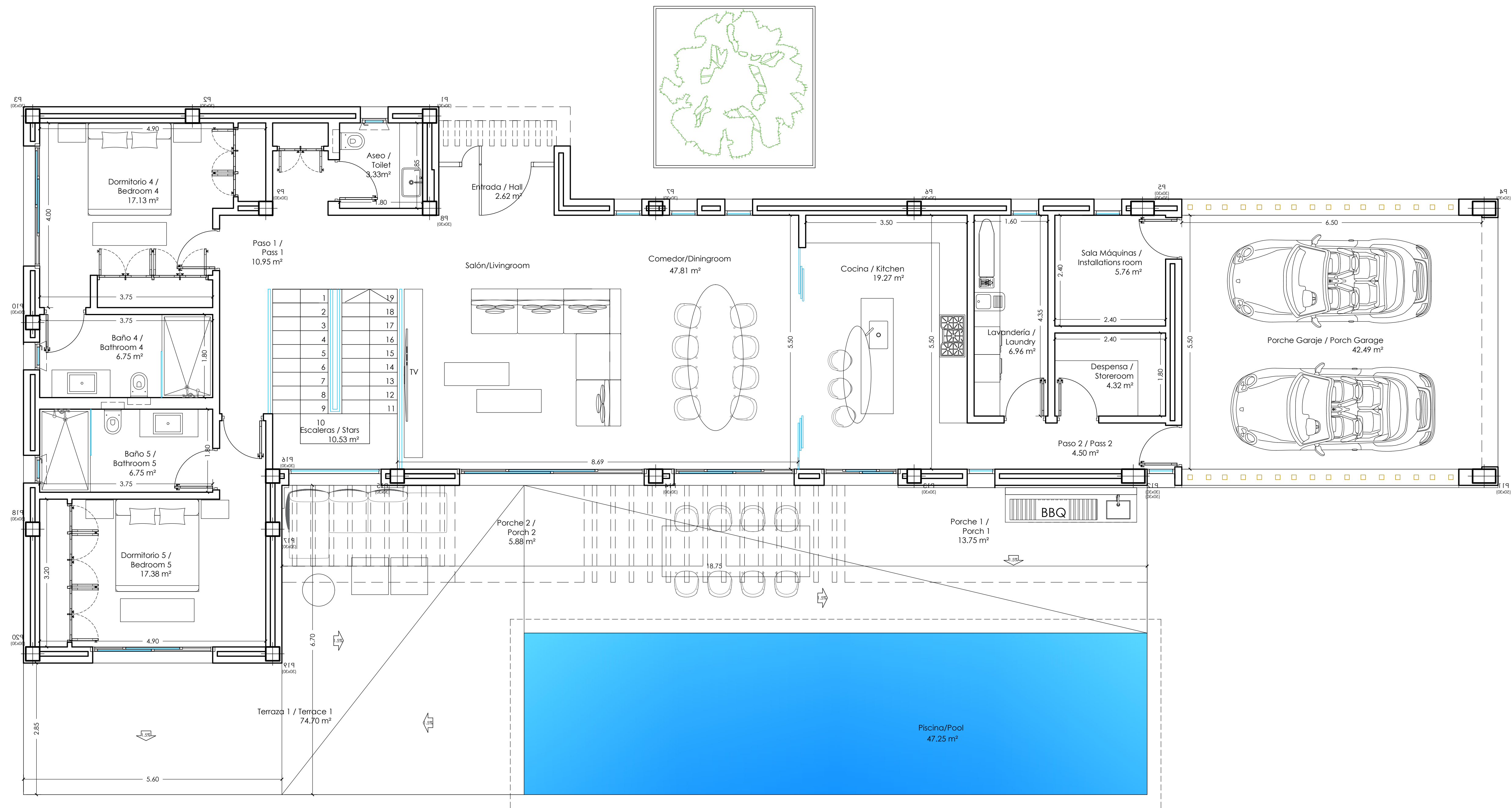
Planta Baja 198.45 m²
