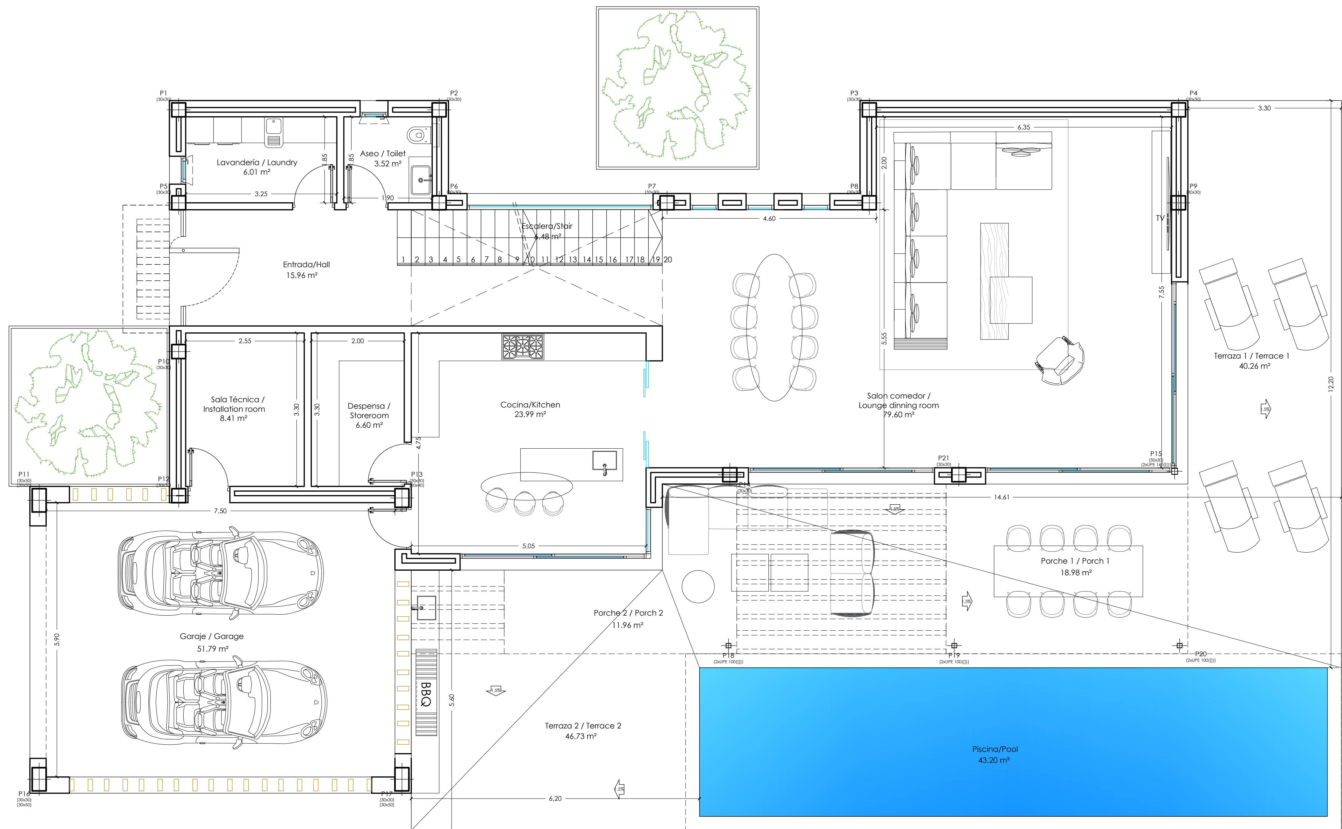
Planta Baja 175.54 m²
