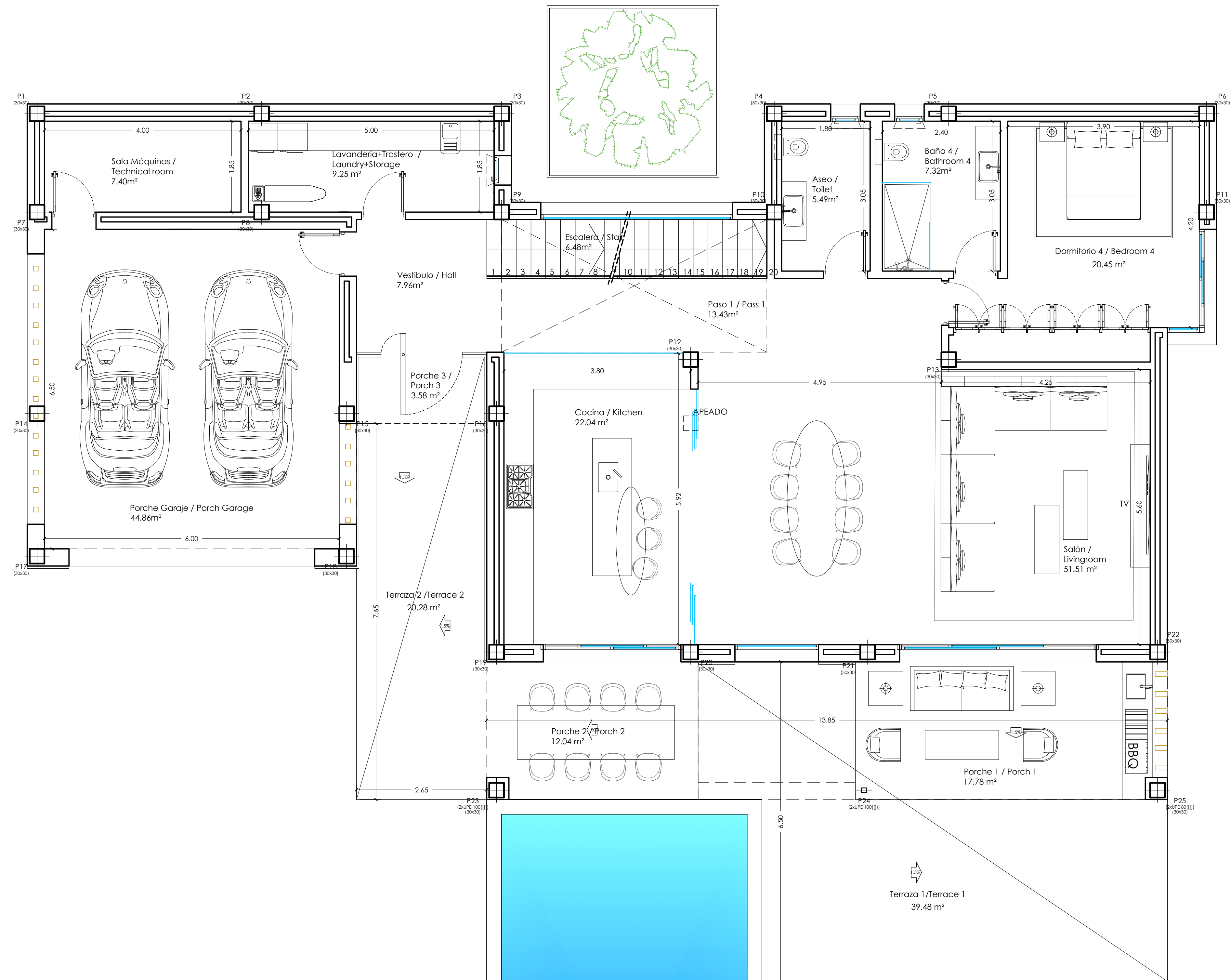
Planta Baja 183.11 m 2
