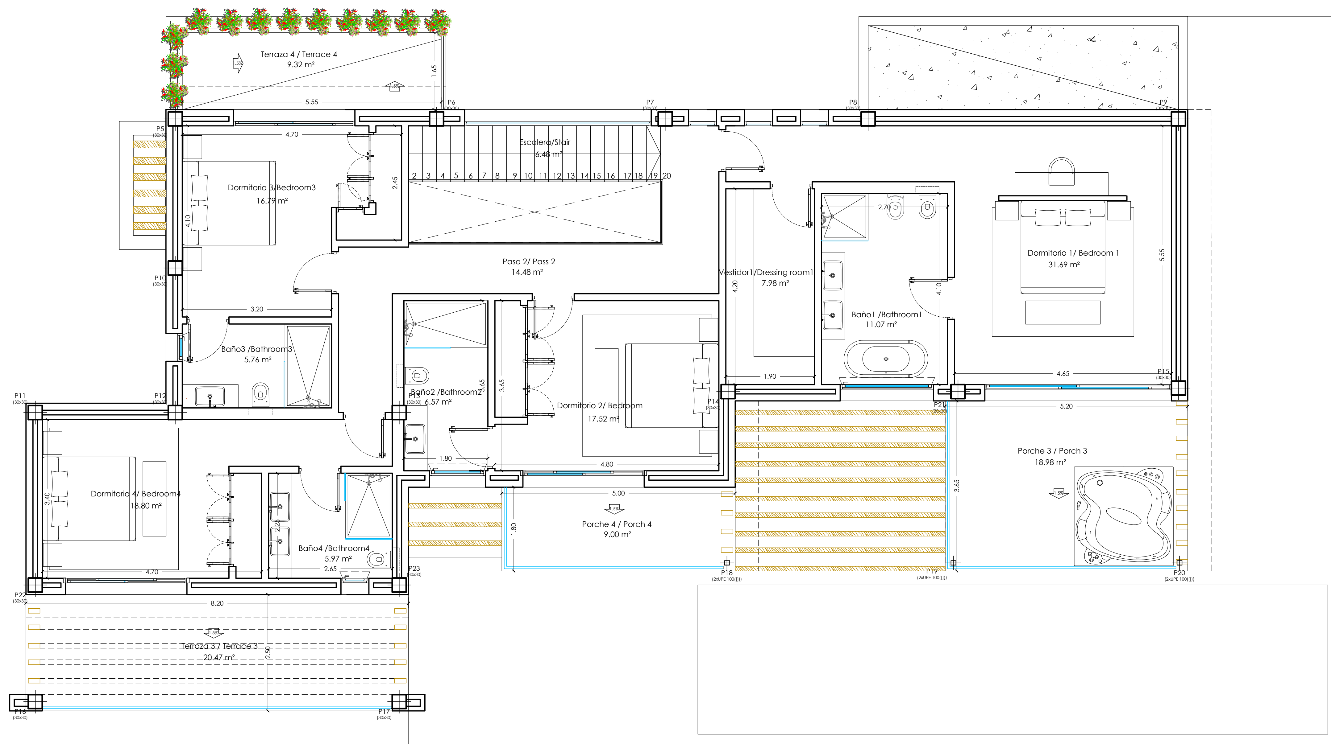
Planta Alta 183.72 m²
