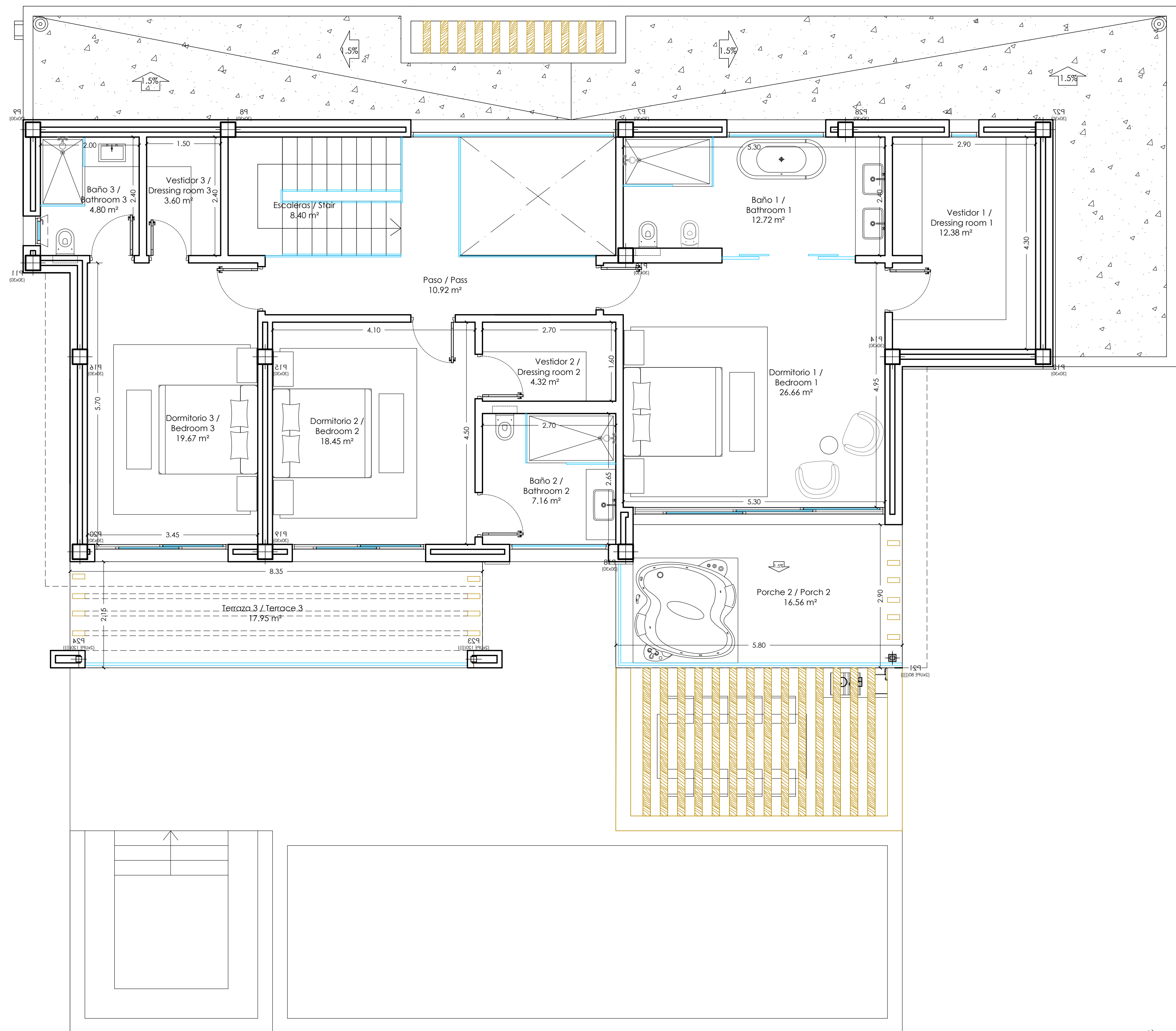
Planta Alta 164.92 m²
