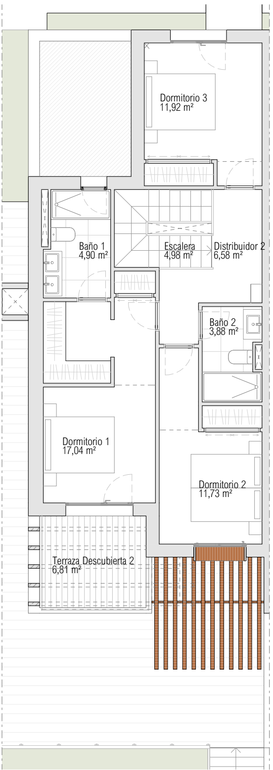
PLANTA ALTA
