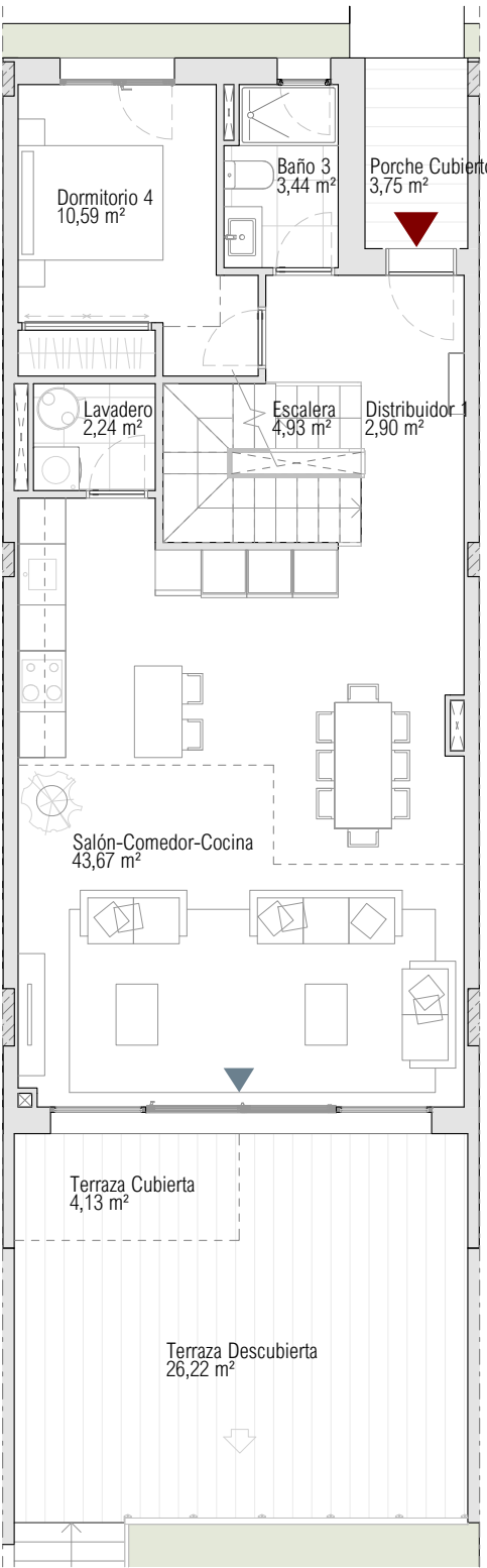
PLANTA BAJA
