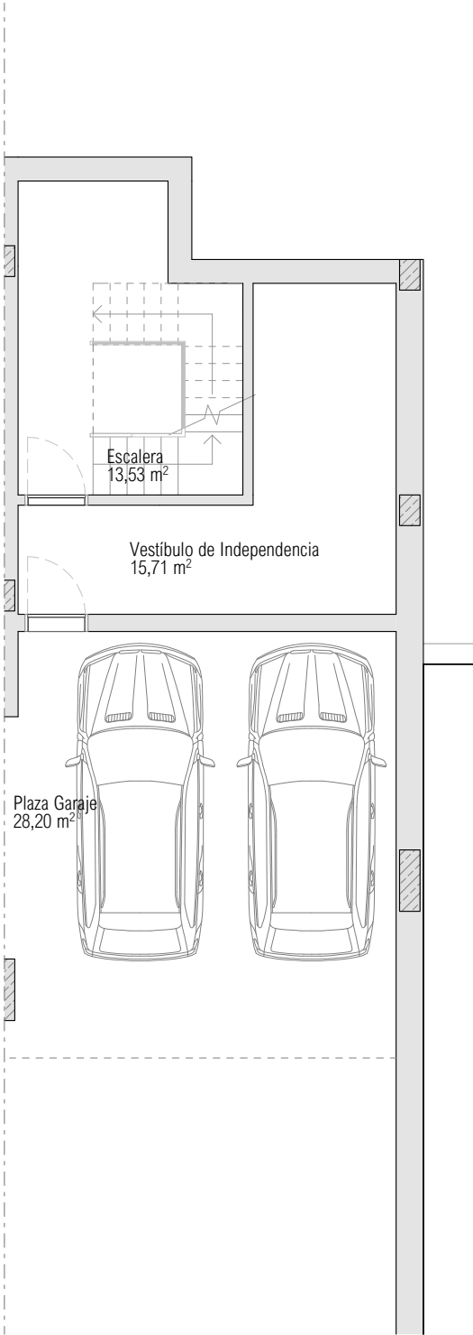
PLANTA SÓTANO
