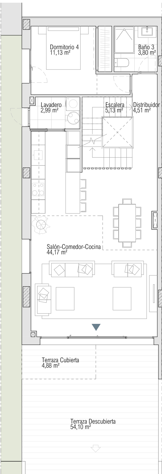
PLANTA BAJA
