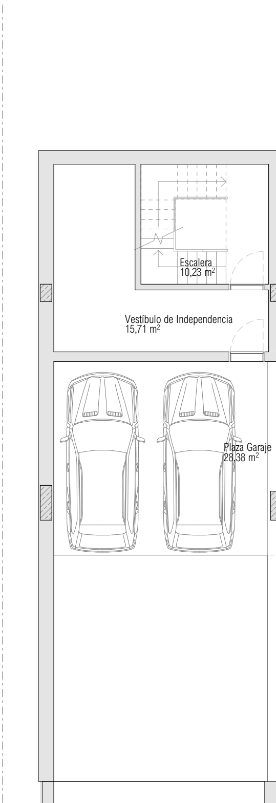
PLANTA SÓTANO
