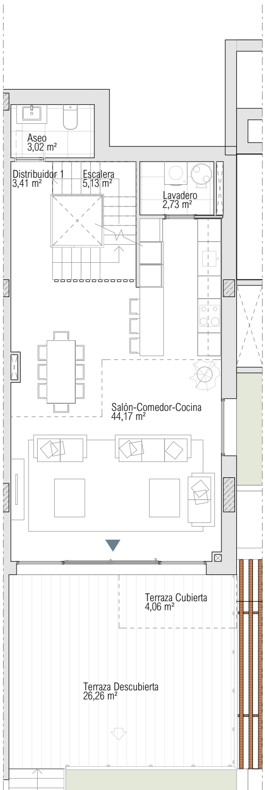
PLANTA BAJA
