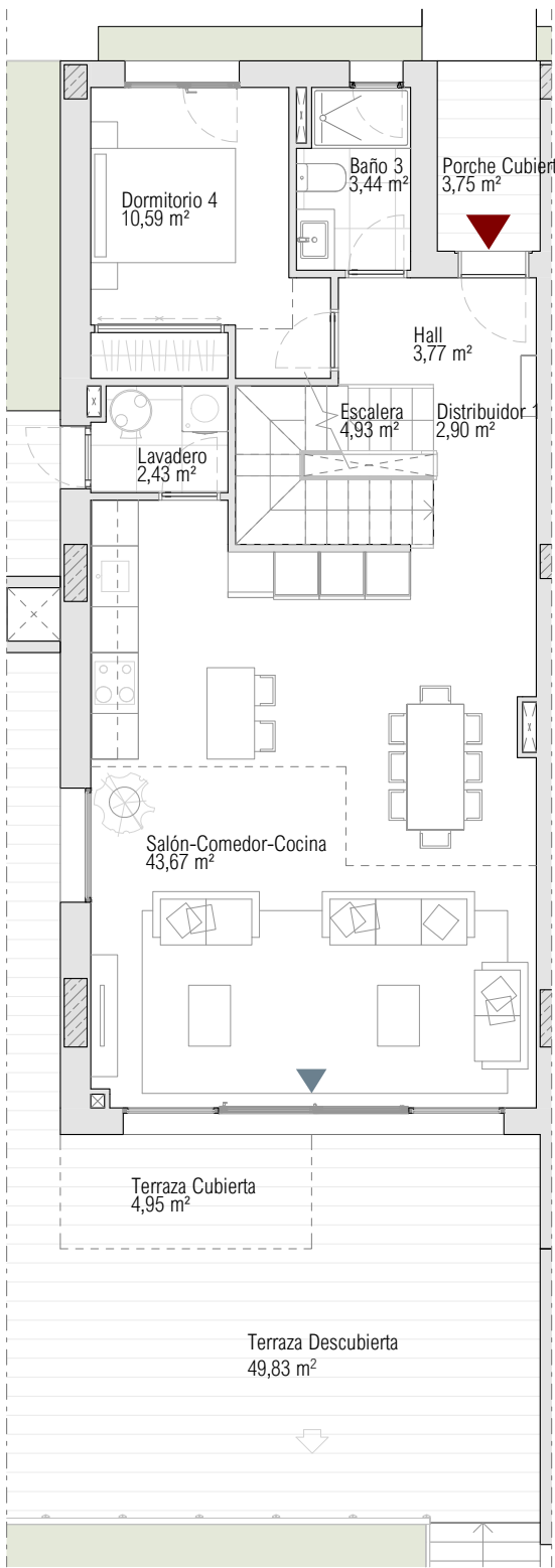
PLANTA BAJA
