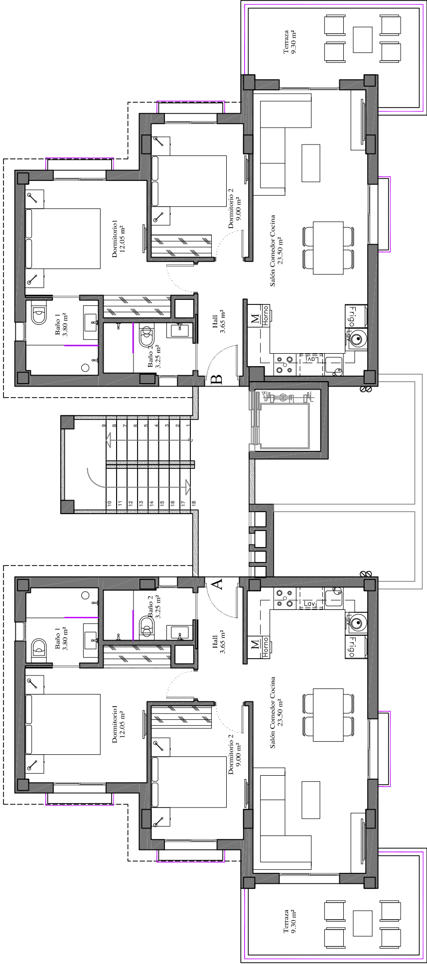
PLANTA TERCERA
