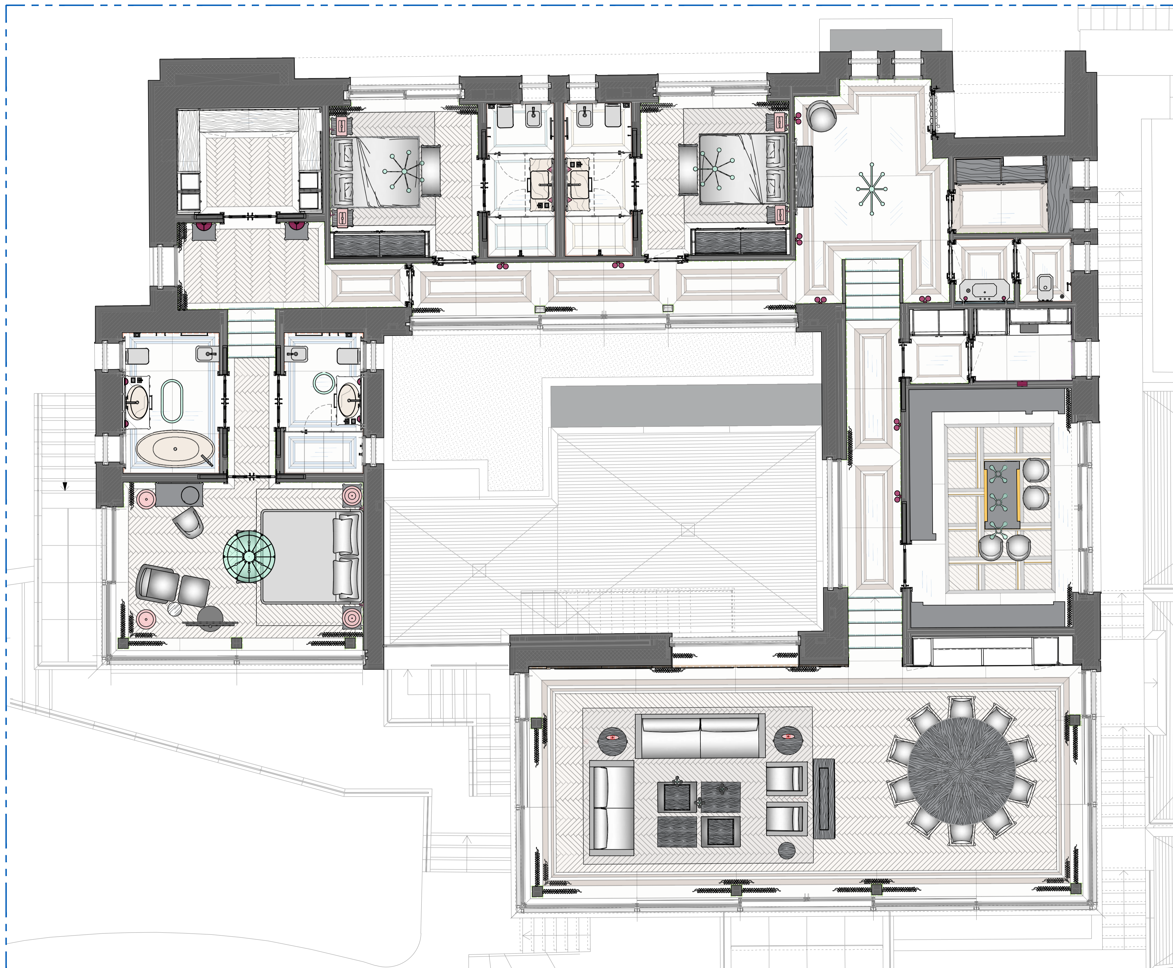
PIANTA SCALA 1:50
