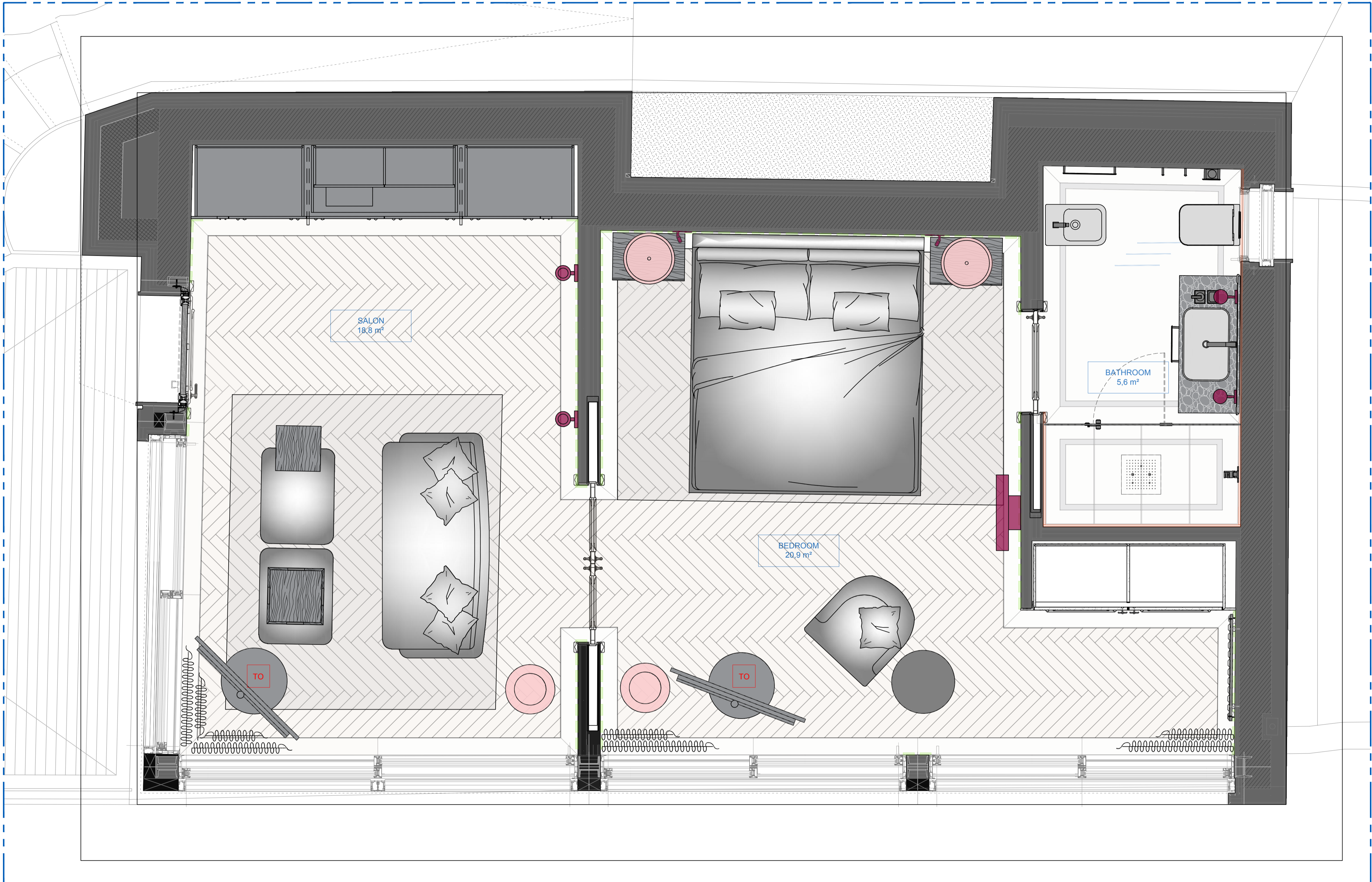
A PIANTA SCALA 1:50
